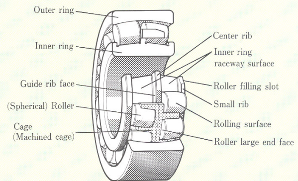
(d) Spherical roller bearing
